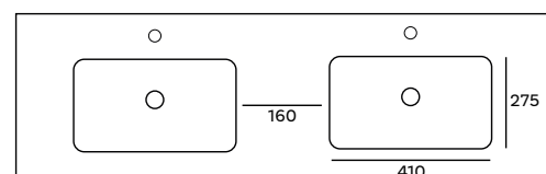
Esquema 120 (2S)
